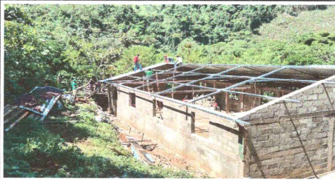
Foto 2: Depues de realizar el desmonte de las vigas de madera y la limpieza general , se procedio a la colocacion de la estructura metalica nueva.
